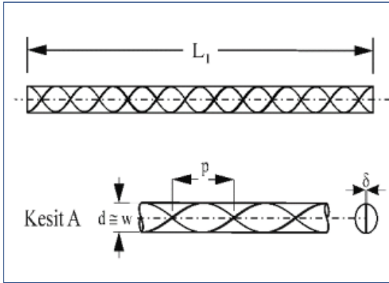
Şekil 4. Burgulu türbülator boyutları
