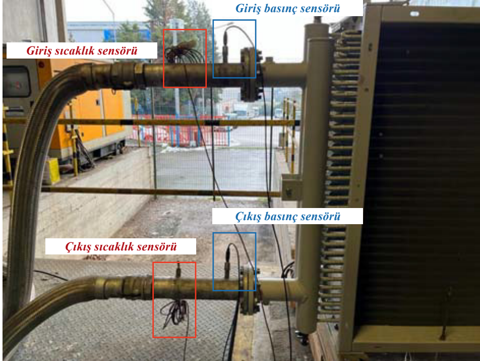
Şekil 8. Akışkan giriş ve çıkış sensörleri
