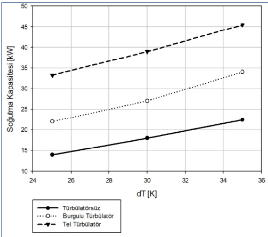
Şekil 11. \Delta T 'ye bağlı olarak türbülatorlerin soğutma kapasitesine olan etkisi
