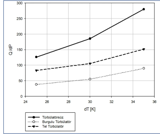
Şekil 12. Birim basınç kaybına düşen kapasite
