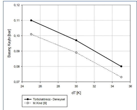
Şekil 9. Sıcaklık farkına ( \Delta T ) bağlı akışkan basınç kaybı değişimi
