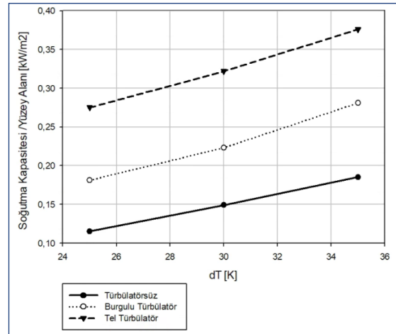
Şekil 13. Birim yüzey alanına düşen kapasite
