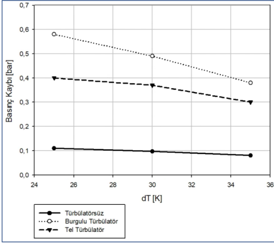
Şekil 10. Farklı tip türbülatorlerin sıcaklık farkına ( \Delta T ) bağlı basınç kaybı değişimi
