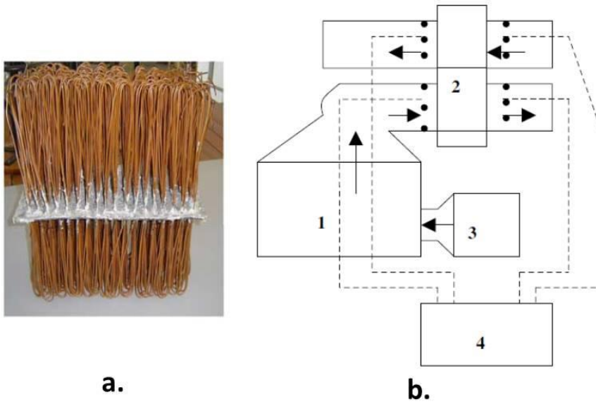
Şekil 6. Isı Borusu Kümesi (a), Deney Düzeneği (b) 1. Kurutucu, 2. IBID, 3.Brülör, 4. Veri Toplayıcı, Isıl çiftler) [7]
