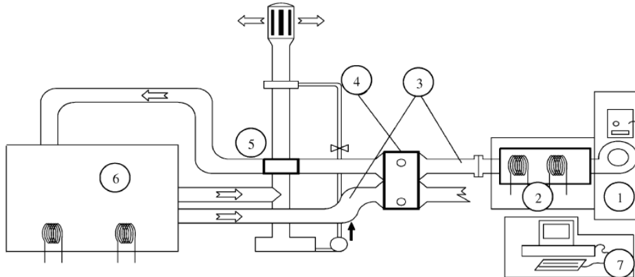
Şekil 10. IBIGK'nın indirek evaporatif IĞK ile kullanımının incelenmesi, 1-2. Klima santrali (İstenilen dış ortam havasını oluşturmak için), 3. Hava kanalları, 4. IBIGK, 5.İndirek evaporatif IĞK, 6. Oda, 7. Veri Toplayıcı sistem [20]
