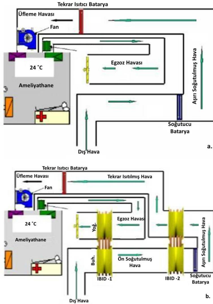
Şekil 16. Mevcut (a) ve İki Adet TIBID Eklenmiş (b) Sistem [22]
