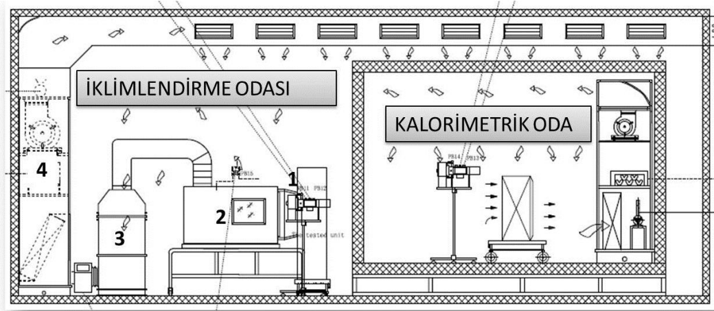
Şekil 20. Test Odası (1. Test Edilen Ürün, 2. Hava Alıcı Oda, 3. Hava Debisi Ölçüm Odası 4. Klima Santrali)
