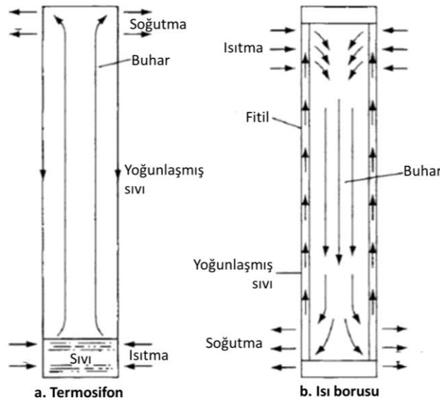
Şekil 1 Termosifon ve Isı Borusunda Akış Şeması [1]
