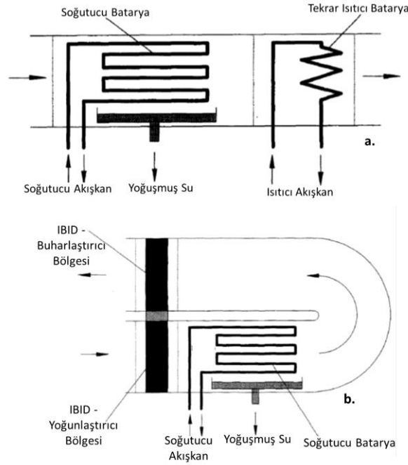
Şekil 15. Tekrar Isıtma Bataryalı (a) ve TIBID (b) Sistem [5]
