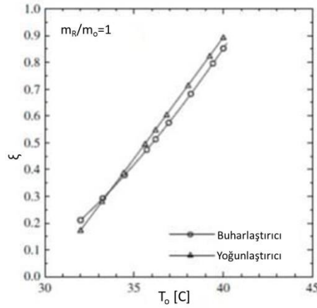
Şekil 9. Taze Hava Sıcaklığının Entalpi Oranına Etkisi [6]
