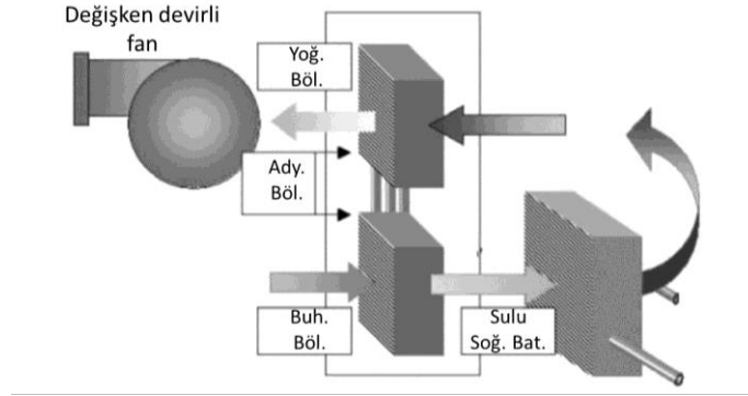
Şekil 7. ÖSTİ için IBIGK-NA Sistemi (Yoğ.Böl.: Yoğunlaştırıcı Bölgesi, Ady.Böl.: Adyabatik Bölge, Buh.Böl.: Buharlaştırıcı Bölgesi, Soğ.Bat.: Soğutucu Batarya) [19]
