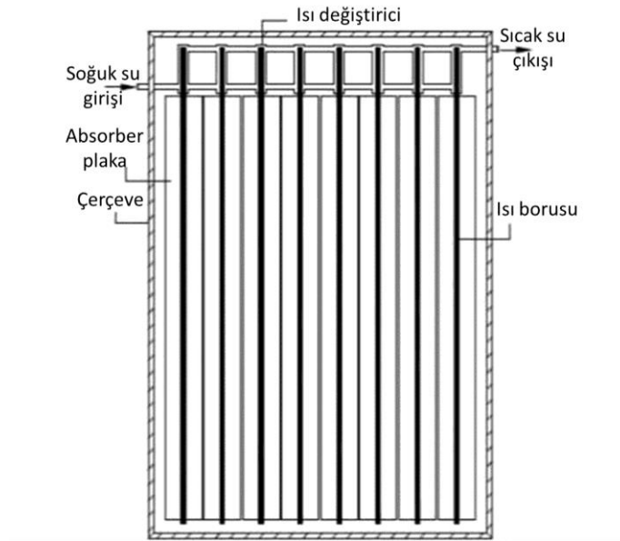
Şekil 5. Güneş Enerjili Su Isıtmada Kullanılan IBID [18]
