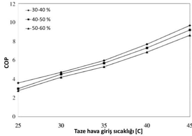
Şekil 11. Taze Giriş Havası Sıcaklığının Farklı Bağıl Nemlerde (HR) Sistemin COP Değerine Etkisi [20].
