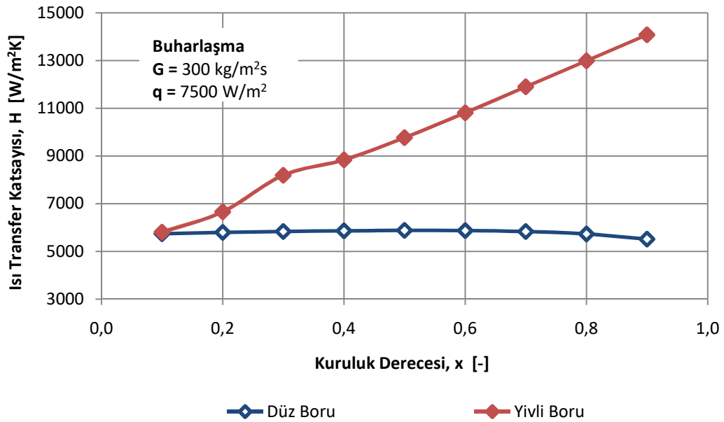
Şekil 16. Farklı kuruluk derecelerinde elde edilen ısı transfer katsayısı değerleri
