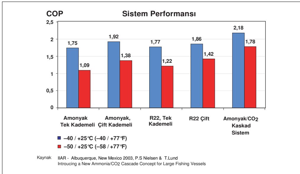
Şekil 12. Farklı sistemlerin COP değerlerinin karşılaştırılması
