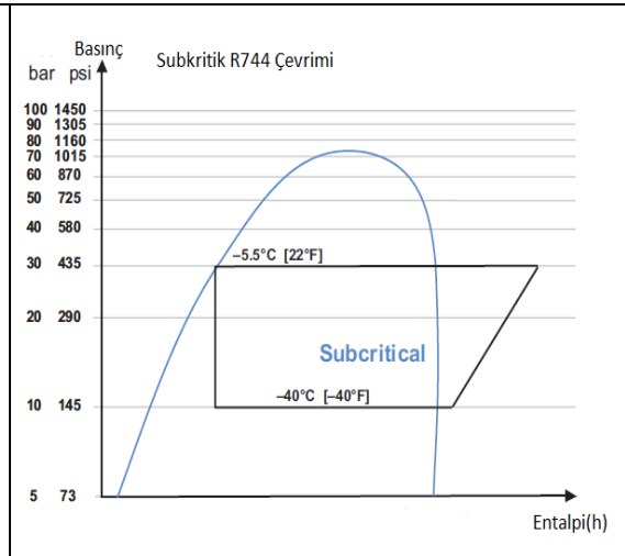
Şekil 4. Direkt Genleşmeli CO 2 Subkritik Çevrim InP - h Diyagramı [10]
