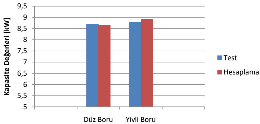
Şekil 20. Test sonuçları ile hesaplamaların karşılaştırılmalı gösterimi
