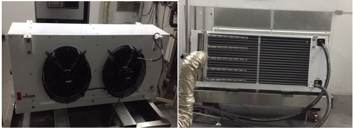
Şekil 17. Kasetli-fanlı buharlaştırıcı prototiplerinin deney düzeneğine montajı
