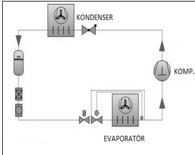
Şekil 3. Direkt Genleşmeli CO 2 Subkritik Çevrim [14]
