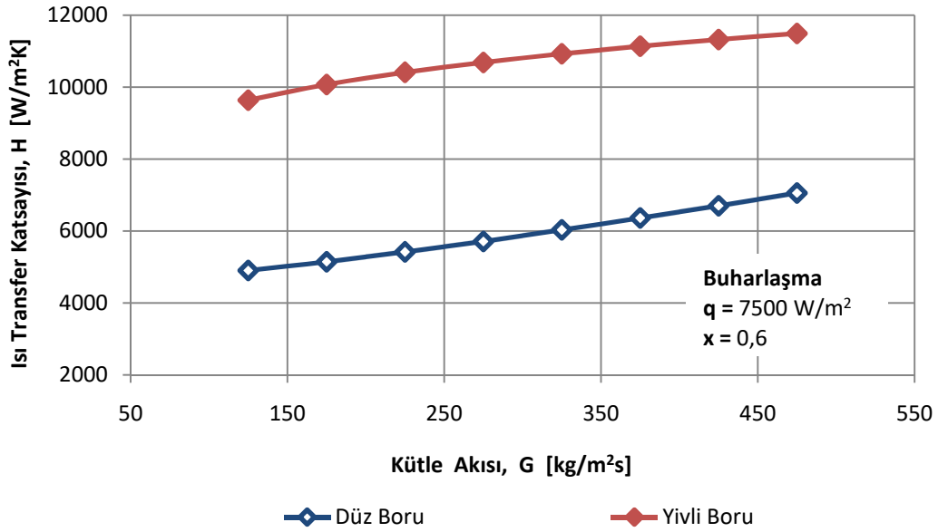
Şekil 15. Farklı kütle akılarında elde edilen ısı transfer katsayısı değerleri
