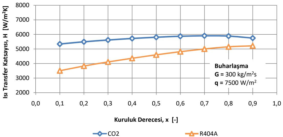
Şekil 14. Farklı kuruluk derecelerinde elde edilen ısı transfer katsayısı değerleri
