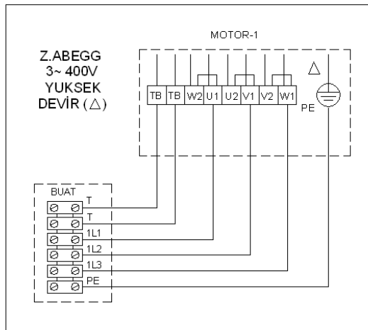
Z.ABEGG 400V Fan Bağlantısı (1 Fan) Z.ABEGG 400V Fan Bağlantısı (2 Fan)
