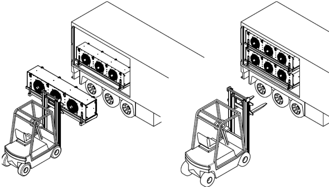
Şekil 1- Taşıma Pozisyonu
