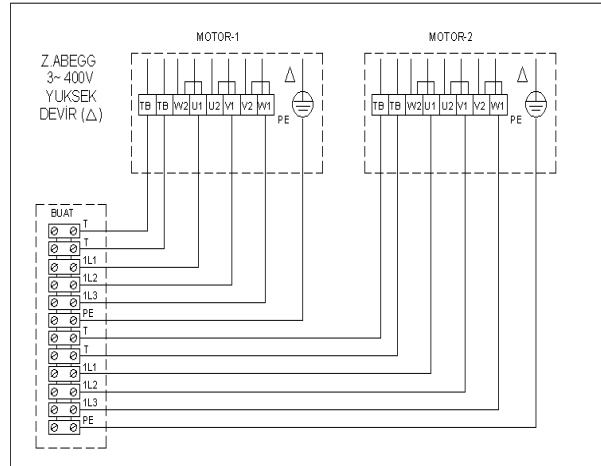
Z.ABEGG 400V Fan Bağlantısı (1 Fan) Z.ABEGG 400V Fan Bağlantısı (2 Fan)
